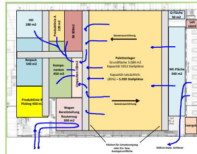
Variante einer Machbarkeitsuntersuchung, Quelle: Projektarbeit SCHÖBER
