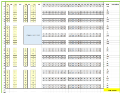
Belegungsplan einer Halle im Maßstab, Quelle: Projektarbeit SCHÖBER
